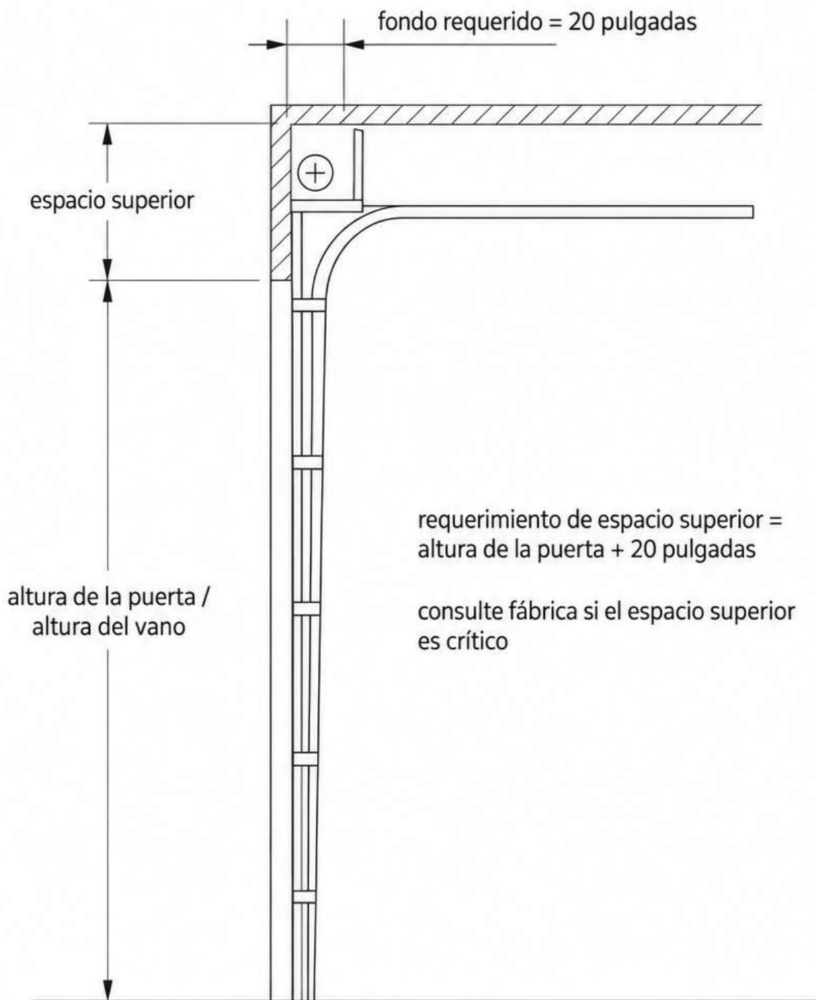
Elevación lateral PB3 / Full Vertical
