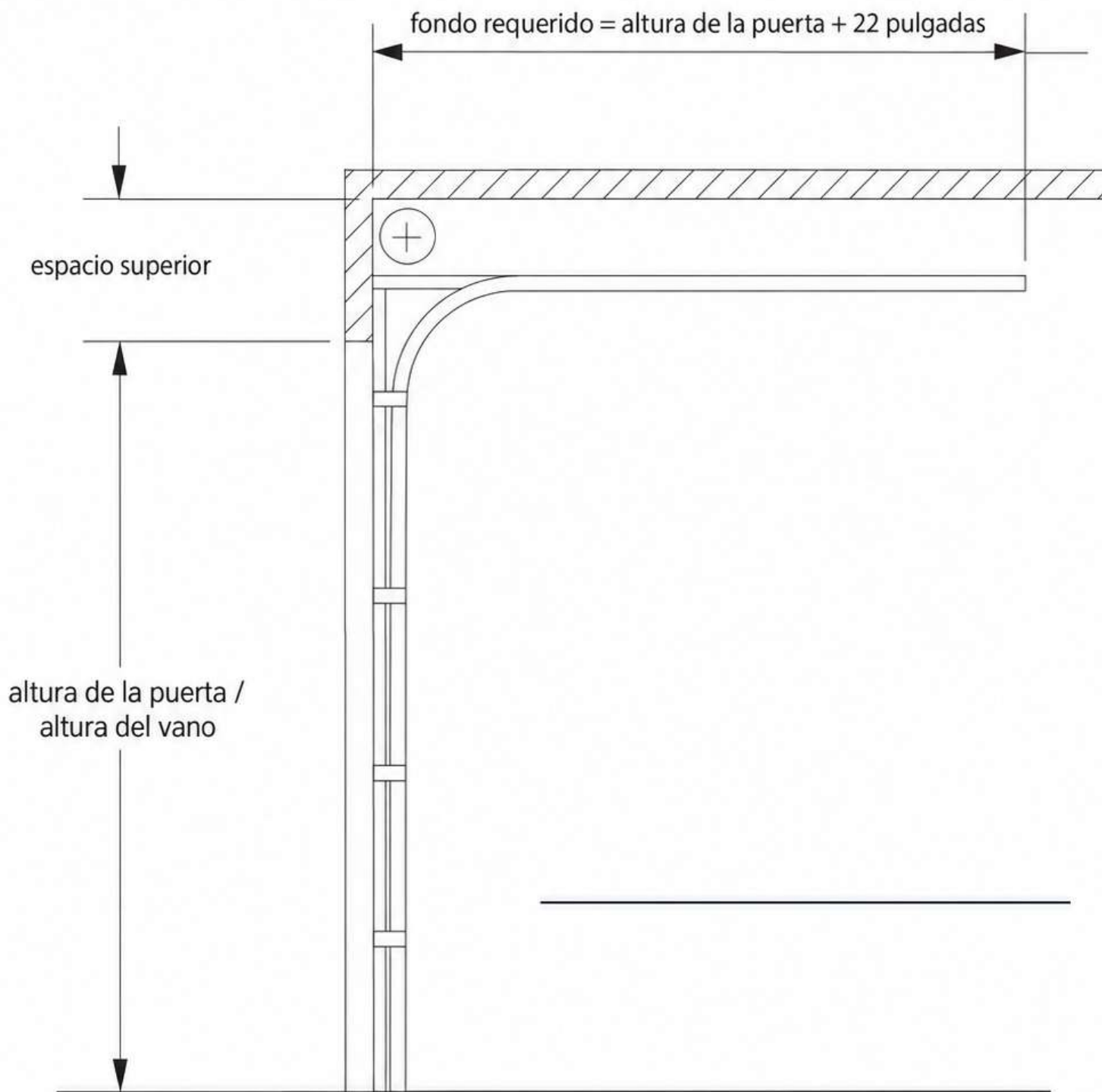
Elevación lateral estándar / Standard side elevation
